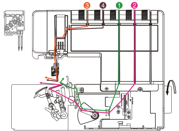
Программа 18 4-ниточный оверлочный шов (R1/ R2)
